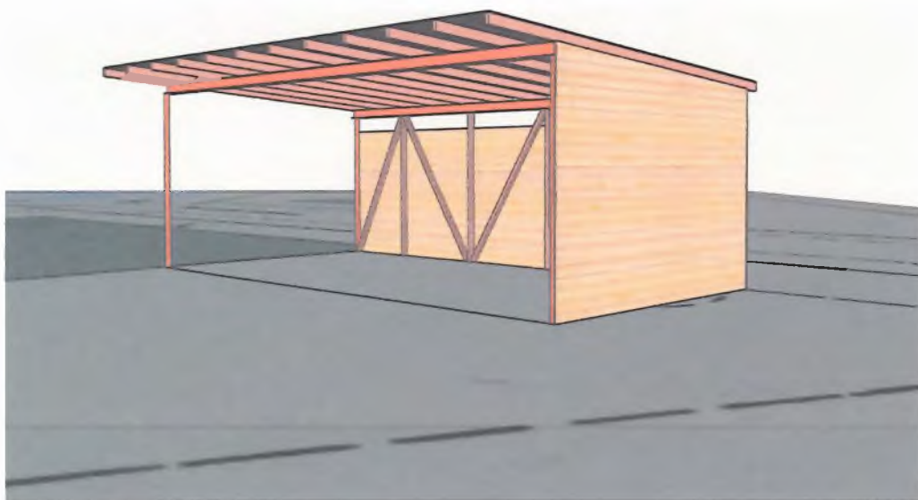
Couvert 1 Longueur: 12m Largeur: 6m Hauteur: 5.2m
