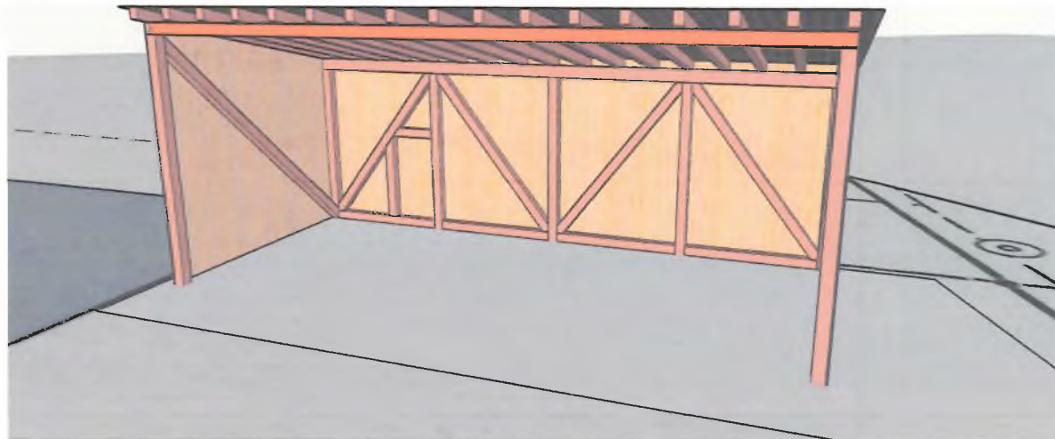
Couvert 3 Longueur: 12m Largeur: 5.5m Hauteur: 6.2
